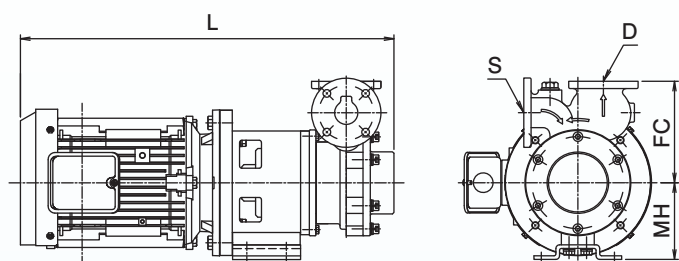
全閉外扇モータ (単位:mm,kg)
